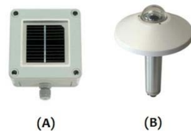
Figura 3. Instrumentos para la medición de radiación solar. (A) Celda fotovoltaica, (B) Piranómetro.
