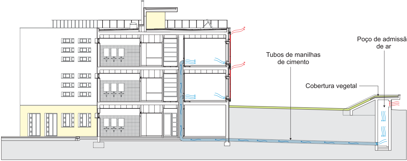
Sistema de arrefecimento do ar através de tubos enterrados
