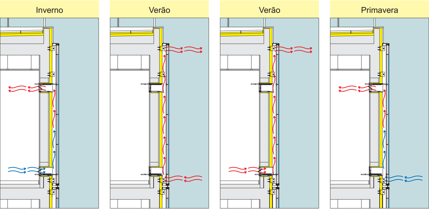
Esquema de funcionamento do sistema fotovoltaico com aproveitamento térmico
