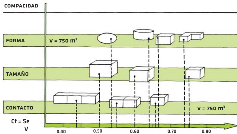
Figura II.1.5.2.1: Variación del coeficiente de forma de un cierto volumen constante.
