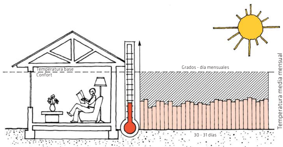
Figura I.3.1.1: Concepto de grados-día
