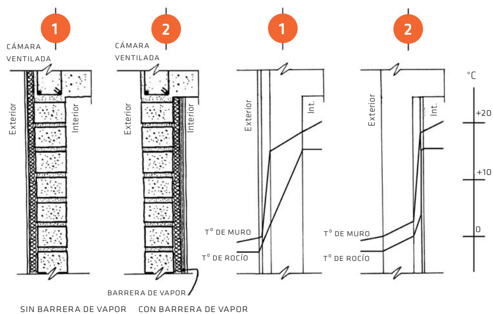
Figura III.3.8.2.4: Riesgo de condensación superficial e intersticial en muro de albañilería con 70mm de aislamiento térmico exterior (1) y 70mm de aislamiento térmico interior (2).
