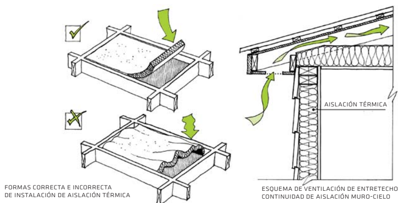
Figura II.1.5.1.2: Aislación térmica bien instalada (izquierda arriba) y mal instalada (izquierda abajo). Caso de aislación térmica bien instalada y continua en encuentro de muro y cielo de la vivienda.
