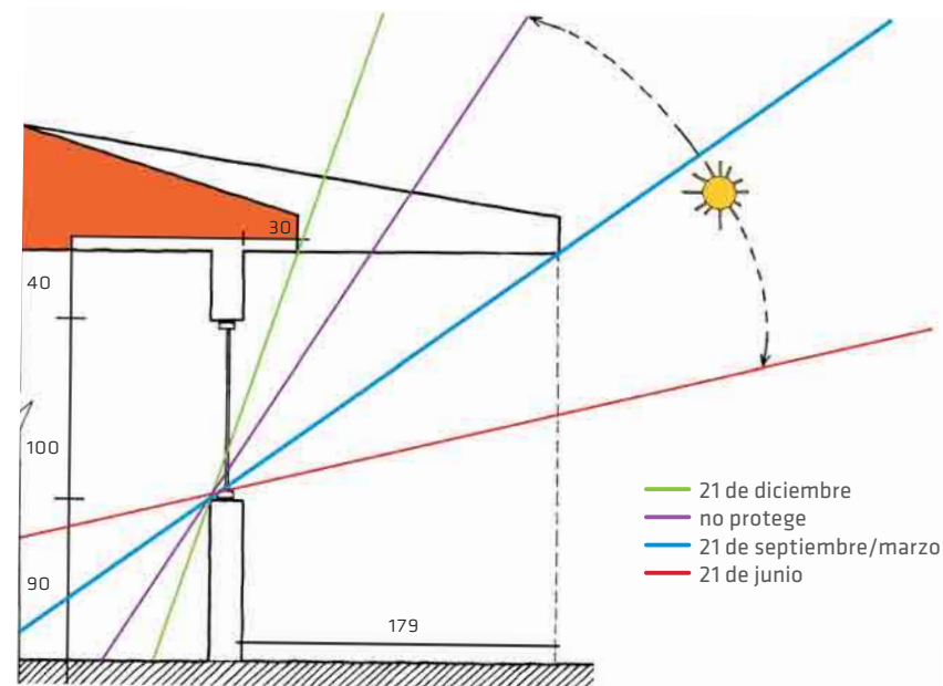
Figura III.3.8.2.3: Dimensionamiento de protección solar horizontal norte para latitud 53° (Punta Arenas)
