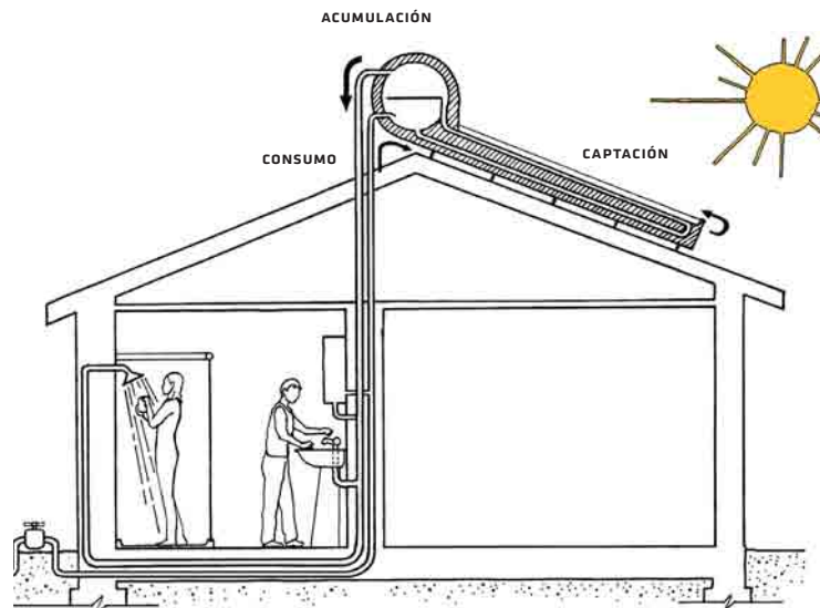
Figura II.3.1.1: Sistemas involucrados en una instalación solar.
