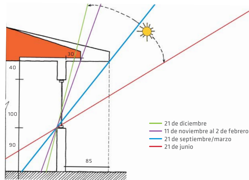
Figura III.3.9.2.3: Dimensionamiento de protección solar horizontal norte para latitud 34° (El Teniente).
