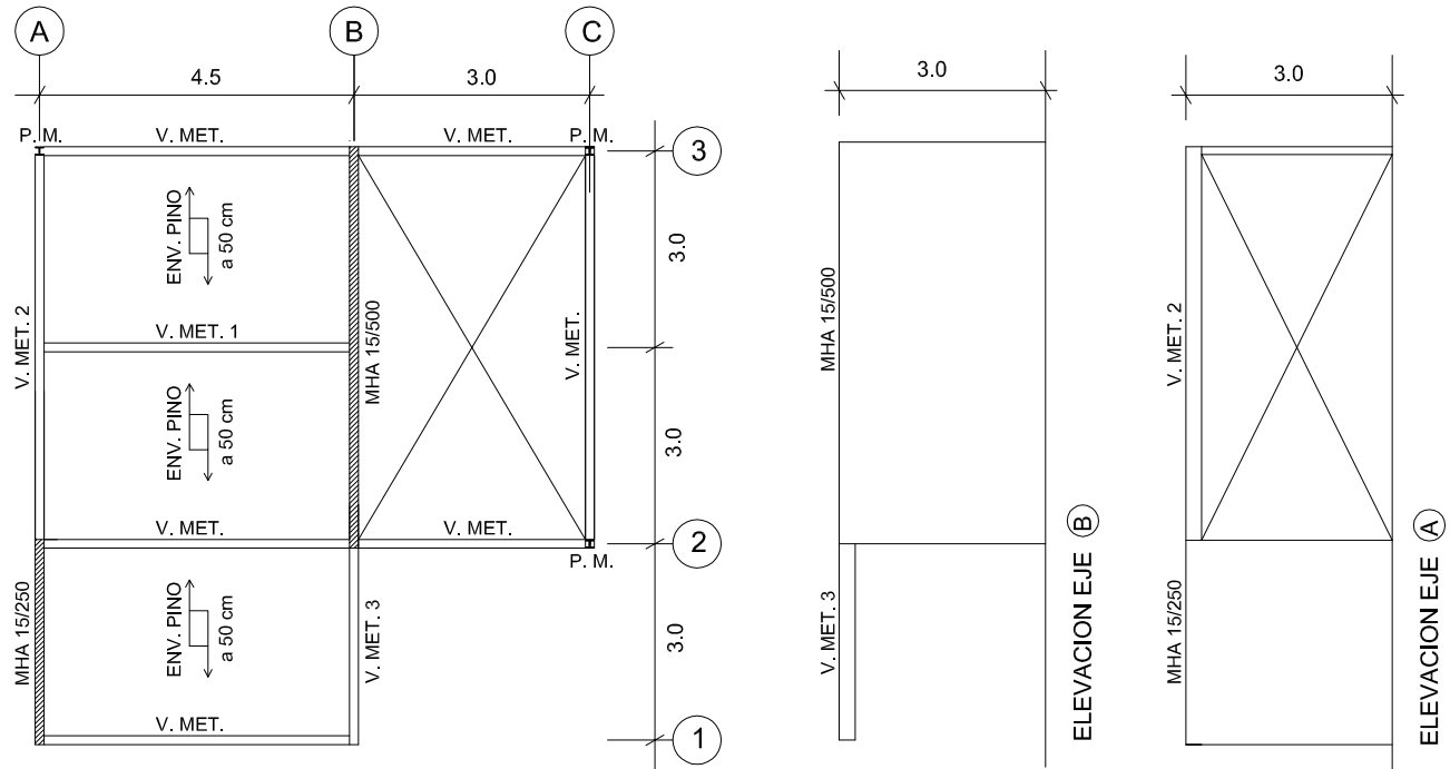
PLANTA ESTRUCTURA
