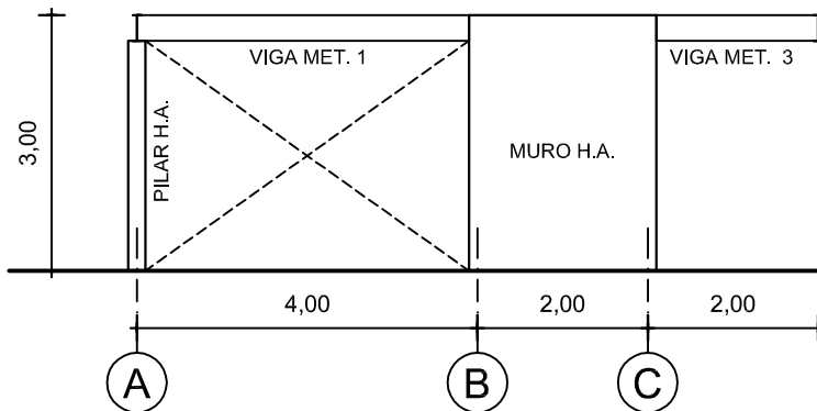
ELEVACION EJE 2
