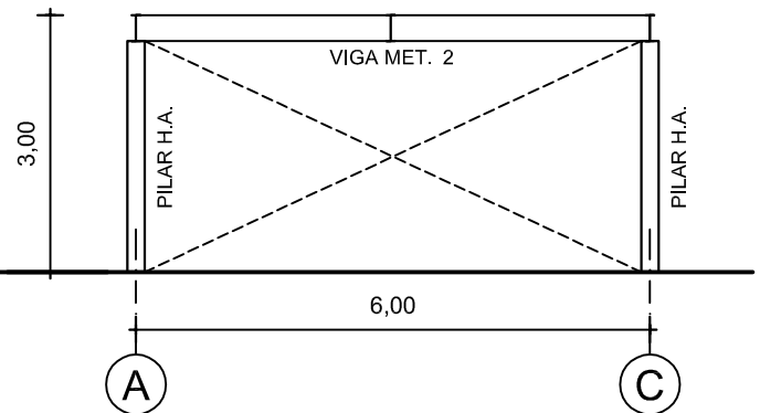
ELEVACION EJE A
