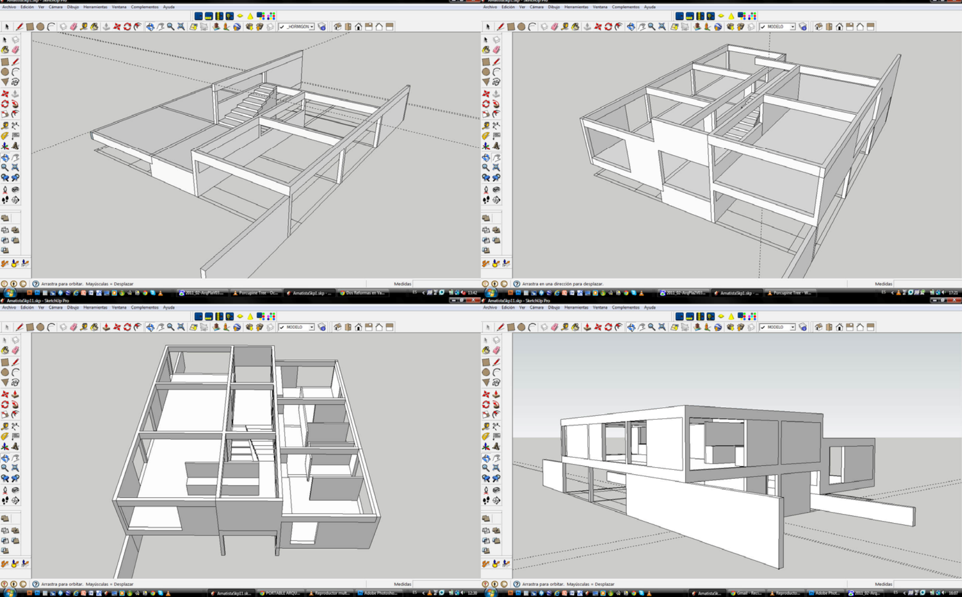
Proyecto de casa en la Reserva. Chicureo ,2011
