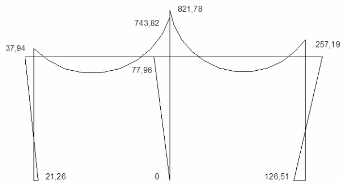
GRÁFICO DE MOMENTOS
