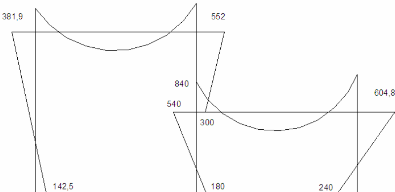
GRÁFICO DE MOMENTOS
