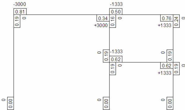
FACTORES DE DISTRIBUCIÓN Y MOMENTOS DE EMPOTRAMIENTO PERFECTO
