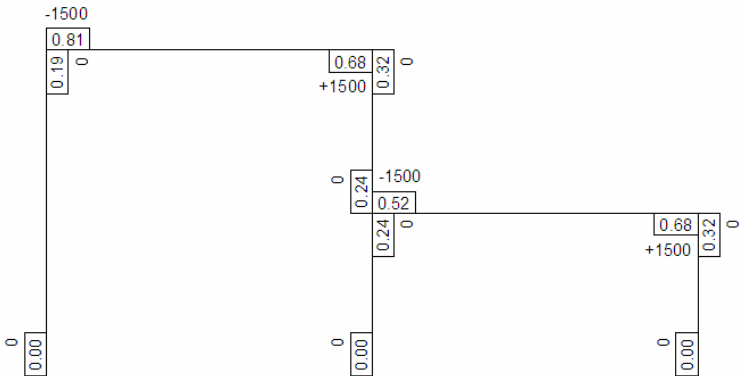
FACTORES DE DISTRIBUCIÓN Y MOMENTOS DE EMPOTRAMIENTO PERFECTO
