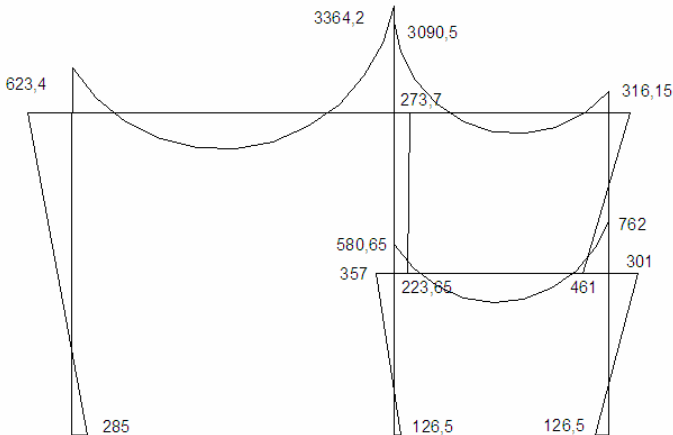
GRÁFICO DE MOMENTOS
