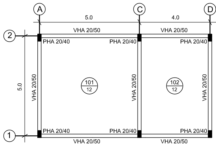
PLANTA ESTRUCTURAS 1º PISO
