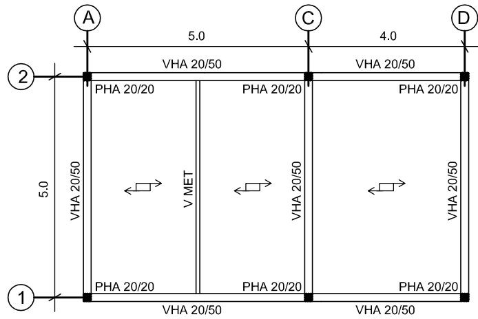
PLANTA ESTRUCTURAS 2º PISO
