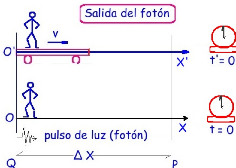
Figura I.5: Salida del pulso de luz (fotón). El origen del sistema de referencia de ambos observadores coincide instantáneamente en t=0=t' . En ese mismo instante se dispara el pulso de luz (fotón). De acuerdo al postulado de Einstein, ambos observadores miden el mismo valor para la velocidad de la luz c . Las coordenadas del punto de llegada es x_P y x'_P en el sistema inercial en movimiento.
