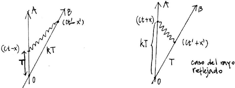
Figura I.44: En la figura de la izquierda debemos identificar T con (ct - x) y kT con (ct' - x') .
