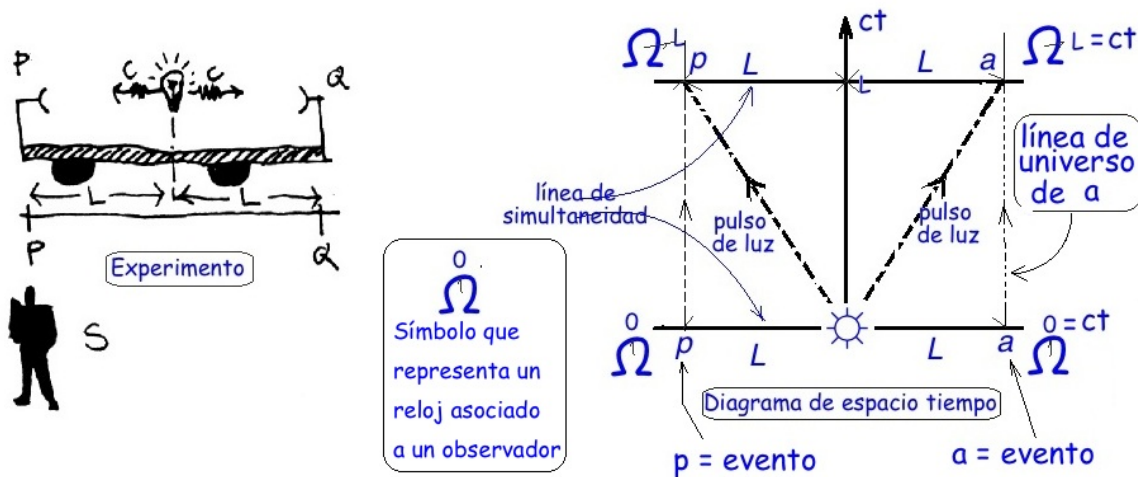
Figura I.16: Dos destellos de luz salen simultáneamente desde el punto medio del carro que se encuentra en reposo en el sistema S . Ambos alcanzan simultáneamente los dos extremos del carro. A la derecha se incluye el diagrama de espacio-tiempo de este experimento.
