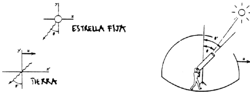
Figura I.36: A la izquierda aparecen los dos sistemas de referencia que están en movimiento relativo. A la derecha se da una idea del cambio de dirección que se le debe dar al telescopio para enfocar la estrella fija (sin movimiento propio).
