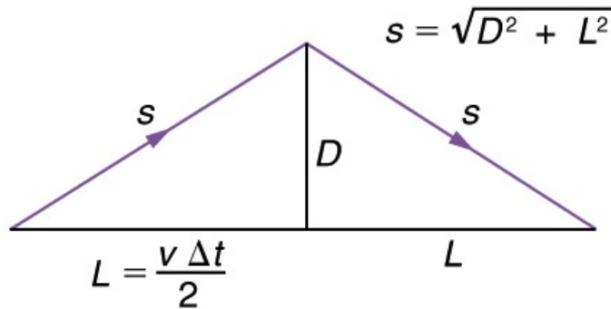
Figura I.27: Geometría de la trayectoria del rayo de luz visto por el observador en tierra.
