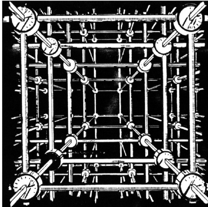
Figura I.19: El observador construye un andamio en su Laboratorio donde cada reloj en cada vértice tiene un tiempo dado por el reloj ubicado allí y también sus coordenadas espaciales. Ambas cantidades fueron asignadas en el proceso de sincronización de cada reloj con el reloj maestro. (Extraído del libro Spacetime Physics , R. Taylor and J. A. Wheeler, W. H. Freeman and Company.)
