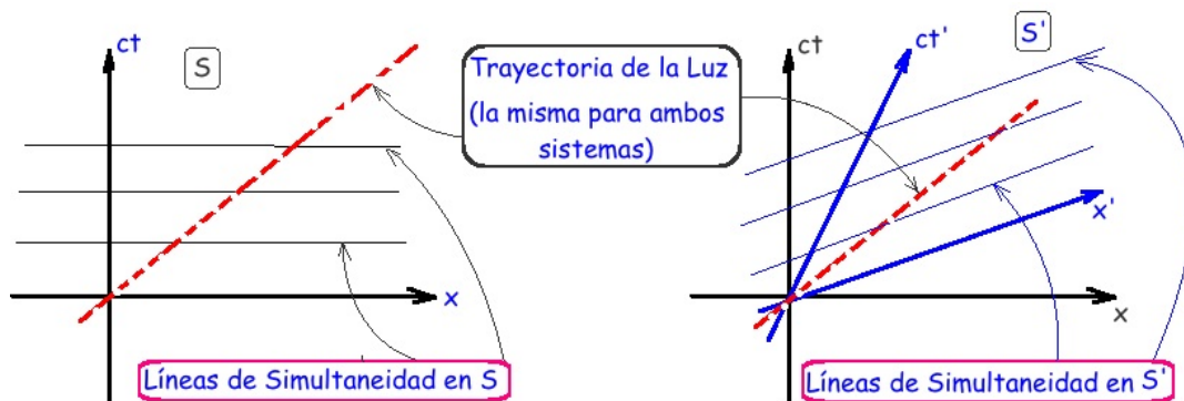
Figura I.18: A la izquierda se dibujan líneas de simultaneidad para el sistema S . A la derecha se ilustra una familia de líneas de simultaneidad en el sistema que consideramos en movimiento relativo con respecto a S , y que denominamos S' . Estas son las líneas construidas en la Figura anterior I.17.
