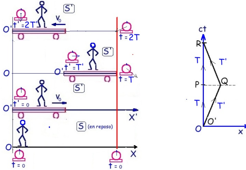
Figura I.25: Diagrama de los gemelos. Uno de ellos emprende un viaje. Al reencontrarse, aquel que fue de viaje es más joven. El quiebre de simetría entre ambos sistemas está en el punto Q de la figura. El gemelo de viaje experimenta una aceleración en esa vecindad y por tanto pierde su carácter de inercial. Los tiempos de ida y regreso mantienen la misma rapidez constante salvo el intervalo con aceleración, y toman el mismo tiempo de viaje por tramo.
