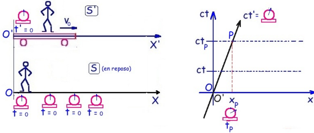
Figura I.23: Las líneas ct y ct' , representan las trayectorias en el espacio-tiempo del origen O y O' de los sistemas de referencia S y S' . P es un punto arbitrario donde se comparan los tiempos indicados por el reloj, fijo en S y ubicado en la coordenada x_P con el reloj fijo al origen de S' .
