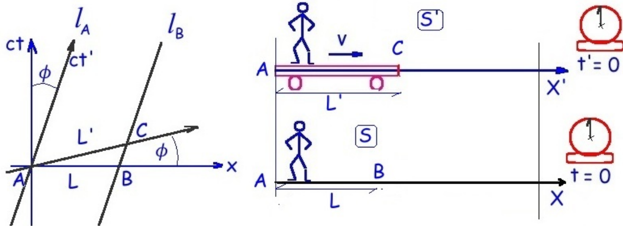
Figura I.21: Las líneas \ell_A y \ell_B , representan la línea de universo (o trayectorias en el espacio-tiempo) de los extremos A y B de la barra rígida en movimiento con respecto al sistema fijo S . El largo definido por el sistema S para la barra es L = \overline{AB} , puesto que es la distancia entre los extremos de la barra y son eventos simultáneos. De la misma forma, L' = \overline{AC} , es el largo definido para la barra por el sistema S' puesto que A y C son eventos simultáneos en el sistema en movimiento S' .
