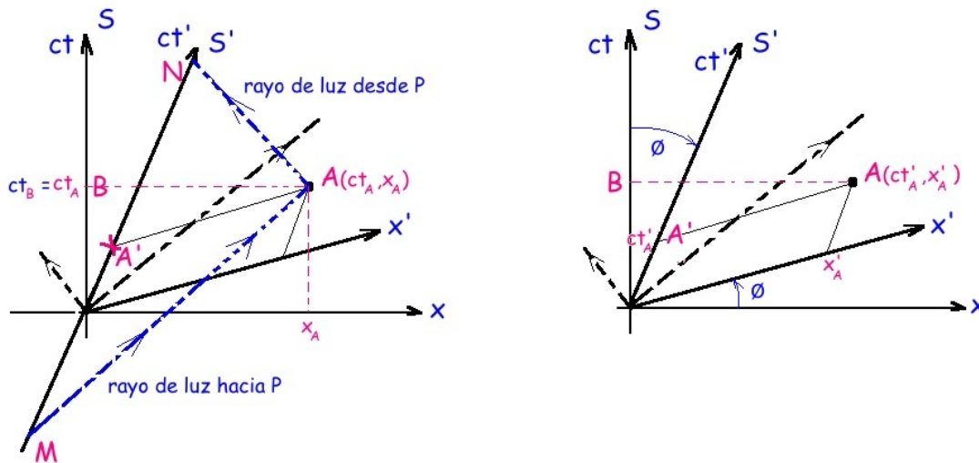
Figura I.20: A la izquierda, se dibuja el rayo de luz que se inicia desde M , rebota en A e impacta en N . De acuerdo al protocolo, el punto medio del trazo \overline{NM} , A' , es el evento simultáneo con A , por tanto para S' los puntos A y A' son simultáneos. Se indican también las coordenadas del punto A en el sistema S (a la izquierda de la figura) y S' . Las coordenadas de A en los sistemas S y S' están relacionadas por las transformaciones de Lorentz [I.2].
