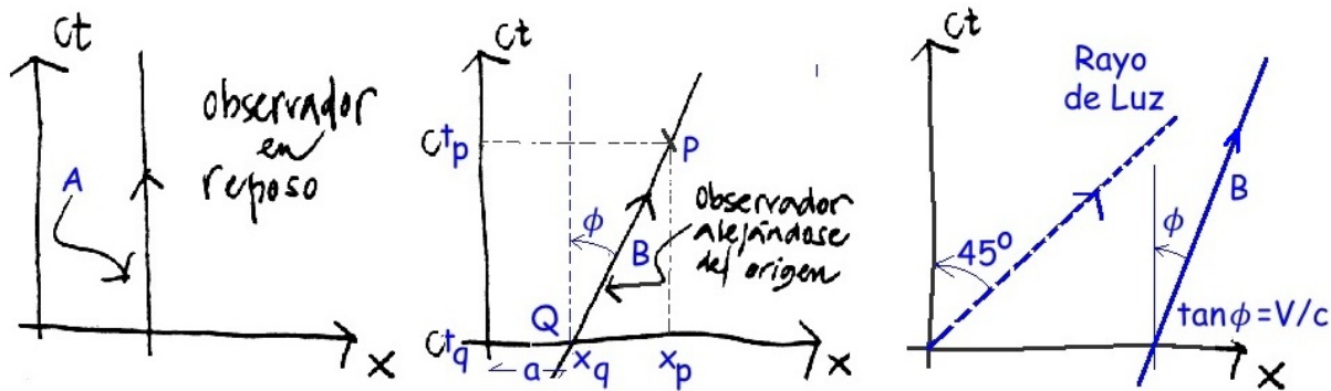
Figura I.8: La línea A, representa la trayectoria en el espacio-tiempo de un observador en reposo en el sistema de referencia. En el diagrama del centro, se dibuja la línea de universo (recta inclinada) de un observador (puntual) que se aleja del origen con una velocidad V . A la derecha se indica la trayectoria de un rayo de luz con su inclinación de 45^\circ y se muestra que \tan \phi = V/c , corresponde a la velocidad del observador B .
