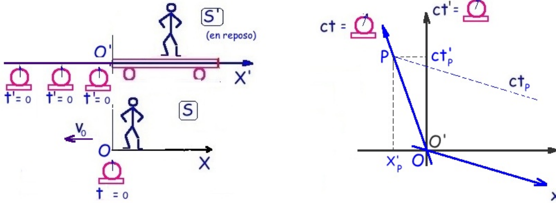
Figura I.24: La línea ct' es vertical porque consideramos a S' en reposo. Ahora es el sistema S se desplaza en el sentido negativo del eje X con velocidad -V_0 . La tangente \tan \phi = V/c es negativa y por eso el sistema de referencia se abre, a diferencia del caso anterior. Se indica una línea de simultaneidad en el sistema S .
