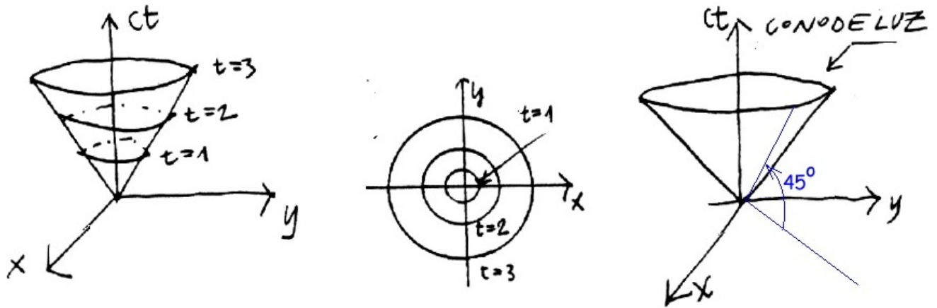
Figura I.7: A la izquierda se dibuja un destello de luz en dos dimensiones espaciales y una temporal. Se representa por un frente circular dibujado en distintos tiempos en la figura. Al centro se dibuja el desplazamiento de esta onda para distintos tiempos, sin incluir explícitamente el eje del tiempo. En la figura de la derecha, el ángulo del vértice del cono es de 90^\circ . Esto refleja que la onda de luz viaja en 45^\circ con respecto al plano de los ejes (x,y) .
