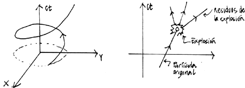
Figura I.9: Línea de universo de una partícula que rota alrededor del origen describiendo una circunferencia de radio a . A la derecha se incluye una partícula que repentinamente explota en tres pedazos. Note que una de las trayectorias es anómala: ¿Cuál parece propagarse con una velocidad mayor que la velocidad de la luz?
