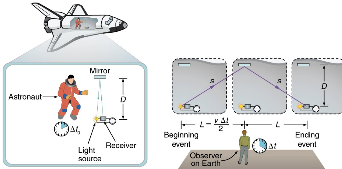
Figura I.26: En el sistema S' , (cohete), el rayo sale y vuelve al origen después de rebotar en el espejo superior. El mismo fenómeno, observado desde tierra permite ilustrar el camino del rayo de luz y la aplicación directa de los principios de la relatividad especial.
