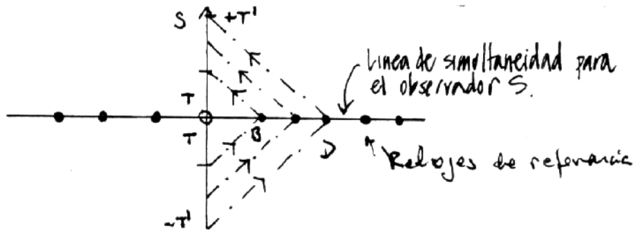
Figura I.14: La luz viaja desde el reloj maestro hasta el punto B , rebota y vuelve al reloj maestro. Demora T segundos en ir y T segundos en volver. El punto medio del intervalo de 2T corresponde al instante cuando el rayo de luz impacta al reloj en B y lo activa. Definimos como simultáneos el instante O del reloj maestro y el evento B . También su distancia queda determinada, es cT .
