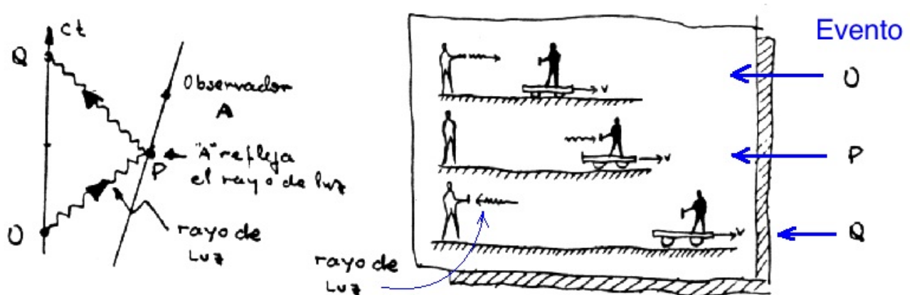
Figura I.11: En la figura de la izquierda, el observador A (en movimiento) recibe un pulso de luz proveniente del observador O (en reposo) y lo refleja de vuelta. En el diagrama de la derecha se representa la misma situación pero como una filmación. En este diagrama el observador A se ubica en el carro que se aleja con velocidad V . Los tres eventos relevantes de la Figura están señalados y son: O, P y Q.
