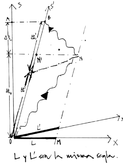
Figura I.39: Qué mide el observador S y qué mide el observador S' . Líneas de simultaneidad en cada sistema de referencia.
