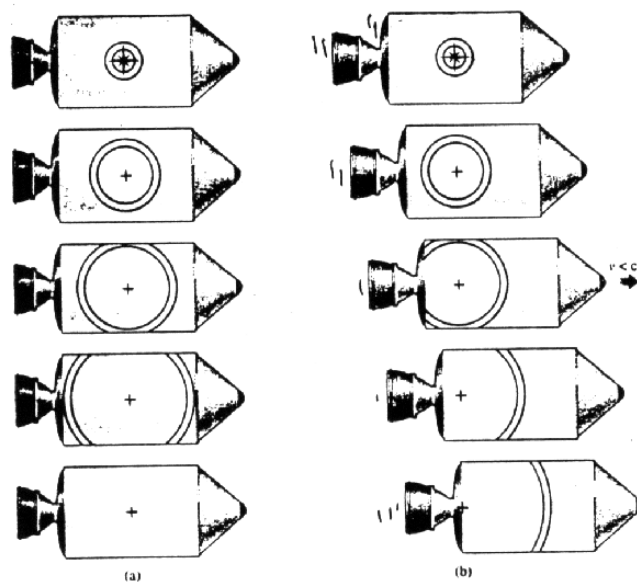
Figura I.28: La propagación de un pulso de luz visto por un observador en reposo en la nave (izquierda, son los círculos concéntricos) y el pulso visto por un observador en reposo fuera de la nave (figura derecha, el centro del círculo permanece en reposo con respecto al sistema de referencia del observador). Para éste el pulso se propaga con la velocidad c y alcanza la cola de la nave antes que la nariz, a diferencia de lo observado por el piloto de la nave.
