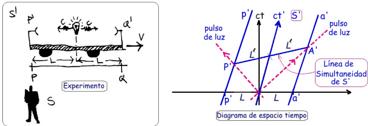
Figura I.17: Dos destellos de luz salen simultáneamente desde el punto medio de la barra de largo 2L' . Esta barra viaja fija al sistema S' . Como se fundamenta en el texto, estos dos pulsos llegan simultáneamente, de acuerdo al sistema S' , en los eventos marcados en la Figura a la derecha, como A' y P' . La recta P'A' es la recta de simultaneidad para S' . Queda claro que la simultaneidad en el sistema S y S' son diferentes. Esta es la definición de simultaneidad relativa, asociada a un sistema de referencia inercial específica.
