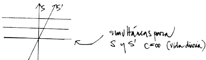
Figura I.13: Los planos de simultaneidad son las líneas horizontales. Son los mismos para todos los observadores inerciales. Si la velocidad de la luz es infinita, nos lleva a la existencia de la simultaneidad absoluta.
