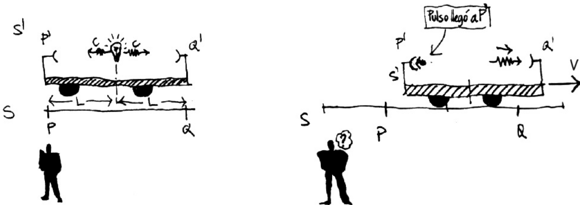
Figura I.15: A la izquierda se muestra el lanzamiento de dos destellos de luz simultáneamente desde el punto medio del carro que se encuentra en reposo en el sistema fijo S . Ambos alcanzan simultáneamente los dos extremos del carro. A la derecha se ilustra el mismo fenómeno, dos destellos de luz que arrancan desde el punto medio del carro en movimiento donde viaja el observador S' . De acuerdo a S , el pulso de la izquierda llega antes puesto que el otro pulso el punto a' se aleja. la velocidad del destello no depende de la velocidad del carro, es una constante universal.
