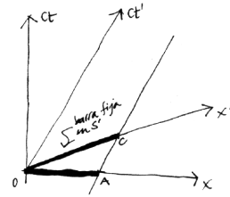
Figura I.35: La figura señala lo que mide el observador S y S'.
