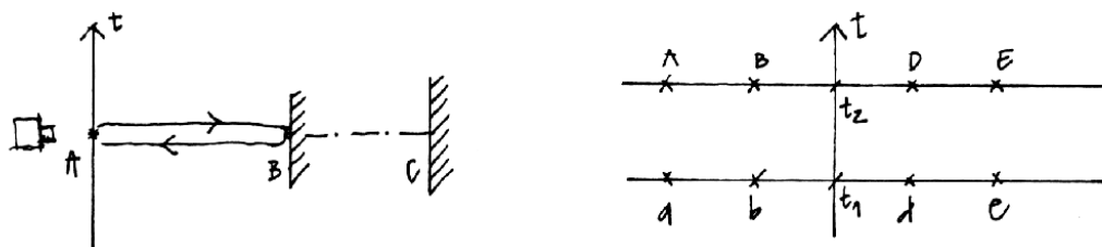
Figura I.12: Un destello de luz viajando con velocidad infinita. Llega a todos los lugares simultáneamente.
