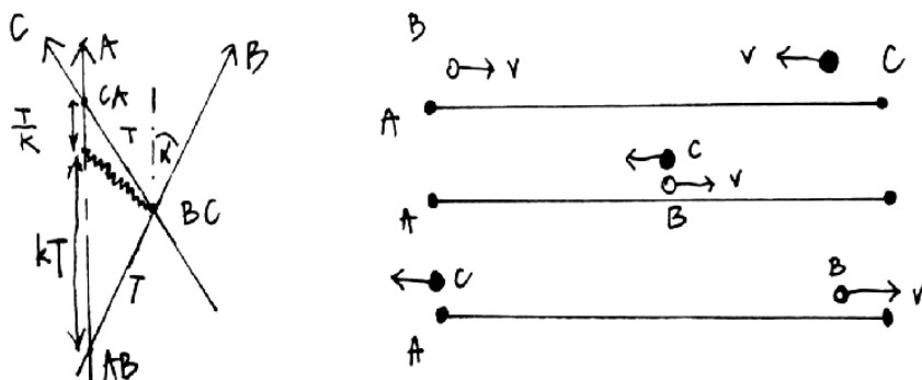
Figura I.40: Nos ubicamos en A, sistema en reposo. B se aleja de A con una velocidad relativa V y C se aproxima hacia A con una velocidad V (según A). A la izquierda se indica el gráfico ct versus x y a la derecha el esquema habitual con la coordenada x en el eje horizontal.
