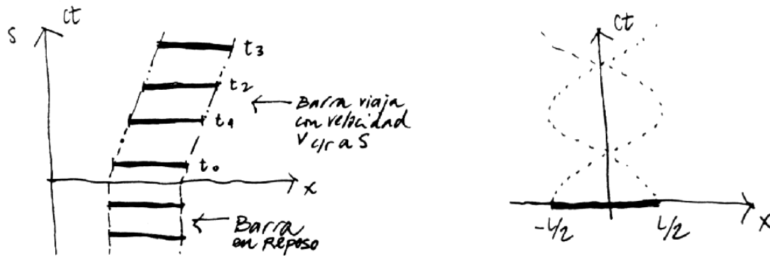
Figura I.10: Línea de universo de los puntos extremos de una barra rígida que permanece en reposo para t \leq 0 y en seguida viaja con velocidad v con respecto al sistema S . A la derecha se indica la línea de universo, proyectada en el plano (ct, x) de los extremos de una barra que gira en torno al origen.
