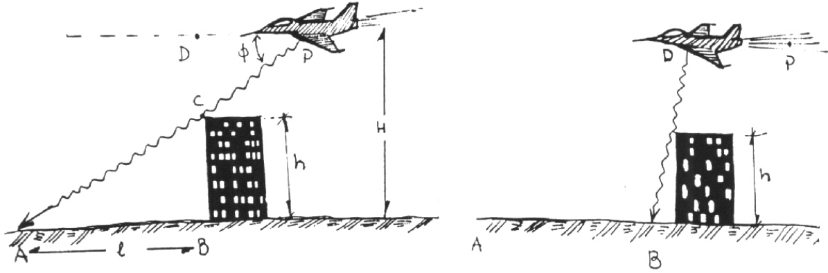
Figura I.45: Al pasar por los puntos P y D el avión enciende una linterna ubicada en cada uno de dichos puntos y que apunta en la forma indicada.
