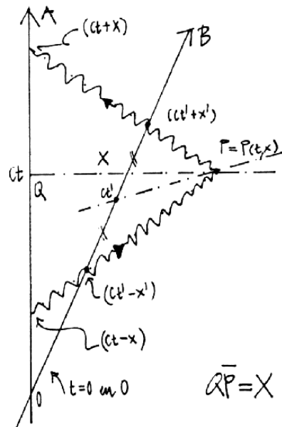
Figura I.43: Un rayo de luz cruza a los dos observadores.
