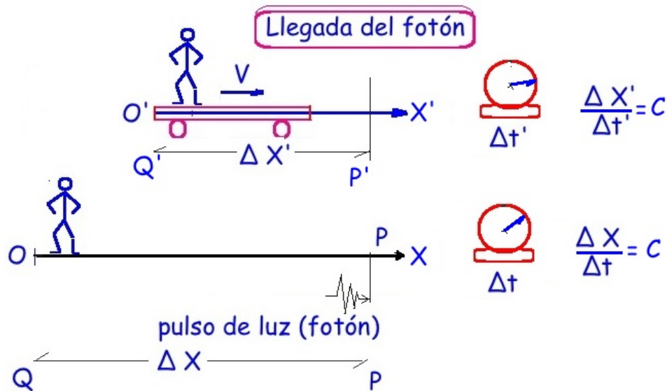
Figura I.6: Llegada del fotón al punto P. Según el observador que dibujamos en reposo, el fotón ha recorrido una distancia igual a \Delta x en un tiempo \Delta t . En el caso del observador en movimiento, la distancia recorrida es \Delta x' medida, como se señala en la figura, a partir del origen de coordenadas de este observador. El tiempo empleado es \Delta t' . El tiempo, como mostraremos más adelante, transcurre en forma diferente en ambos sistemas. La relación entre las coordenadas debe cumplir la condición: \Delta x'/\Delta t' = c = \Delta x/\Delta t .
