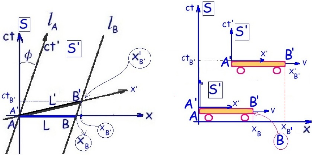
Figura I.22: Las líneas \ell_A y \ell_B , representan la línea de universo (o trayectorias en el espacio-tiempo) de los extremos A y B de la barra rígida en movimiento con respecto al sistema fijo S. A la derecha, el extremo B' medido en el sistema S' es X'_{B'} . Como los eventos B y B' están en la misma línea de universo \ell_B , ambos tienen la misma coordenada en S', o sea X'_B = X'_{B'} .
