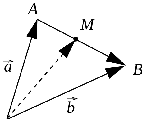
FIGURA 1.10. Punto medio.
