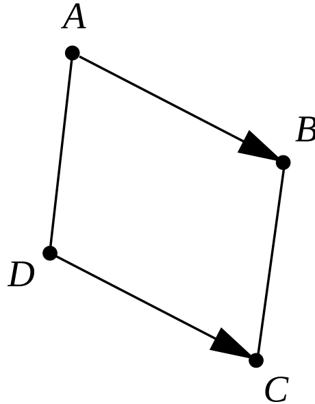
FIGURA 1.3. Paralelogramo.
