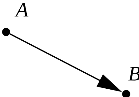
FIGURA 1.2. Vector desplazamiento.
