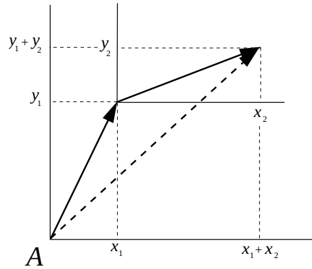
FIGURA 1.6. Suma analítica.
