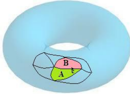
Figure 23.5: Dos s mplices adyacentes en una triangulaci n de una variedad compacta sin borde.
