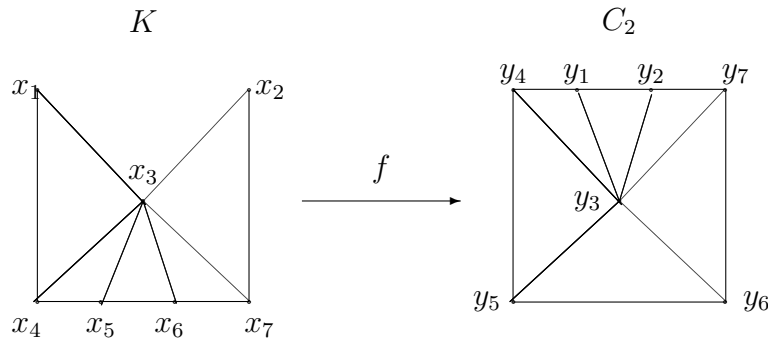
Figure 16.5: Una biyección entre los vértices que induce una función simplicial no epiyectiva..
