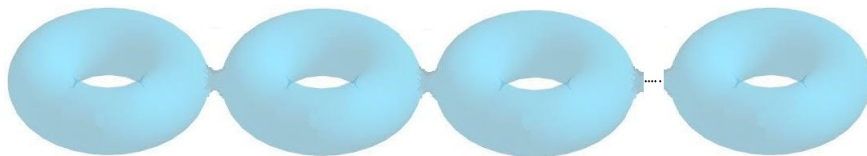
Figure 19.7: La superficie de género g .
