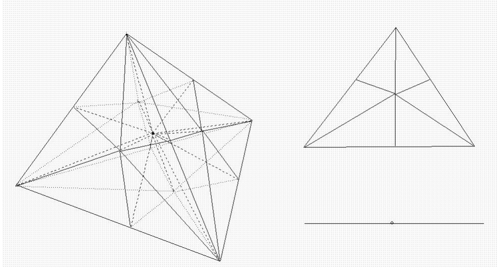
Figure 21.3: Subdivisión batricentrica de símplexes de dimensiones pequeñas..
