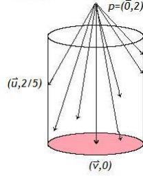
Figure 14.5: Projectando el cilindro en su borde no superior.
