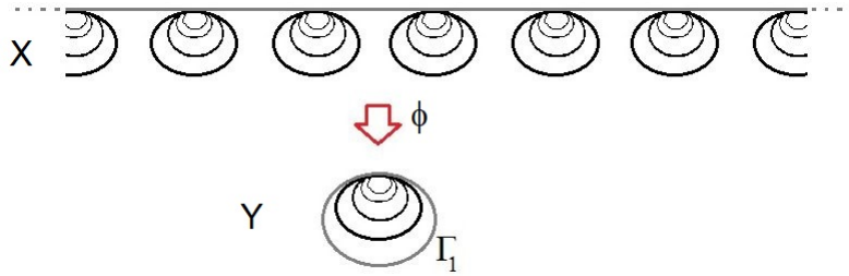
Figure 18.6: El pendiente Hawaiano y un recubrimiento.
