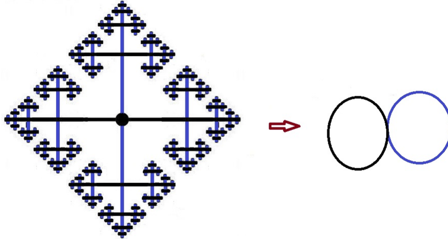
Figure 19.1: La Antena de Televisión universal como recubrimiento de la figura-8 .
