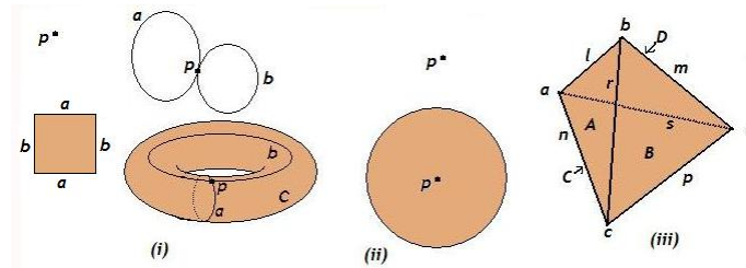
Figure 14.4: Algunos espacios descritos como CW-complejos.
