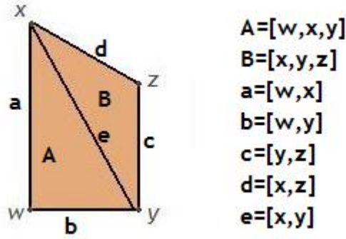
Figure 20.1: Un complejo y una orientación para sus símlices.
