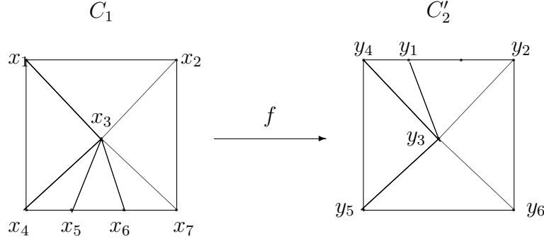
Figure 16.4: Una función simplicial que colapsa un símlice.
