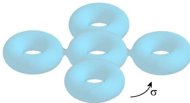
Figure 19.8: Una acción cuyo cociente es el bitoro.
