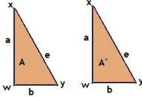
Figure 20.2: Dos s mplices con bordes identificados.
