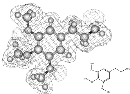
Figura 2.3. PEM de la mescalina neutra. Las isolíneas punteadas corresponden a valores negativos del PEM. Incremento= 0,05.
