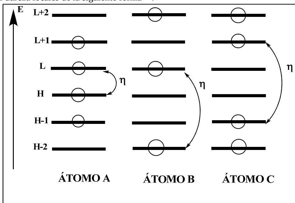
Figure 7.2. Definición directa para el potencial químico electrónico local y la dureza local. Las flechas indican la dureza atómica local como ejemplo.
