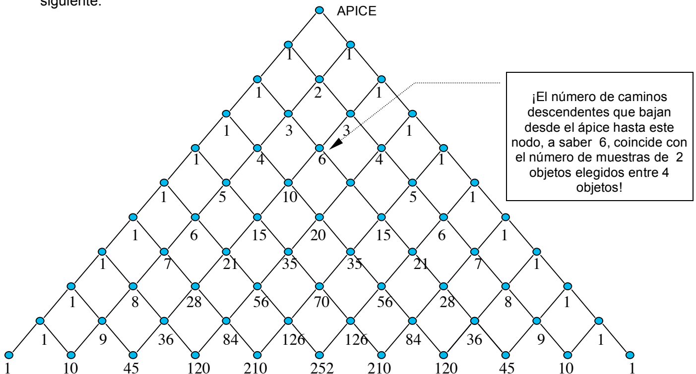
Número de caminos descendentes desde el ápice de una malla triangular
