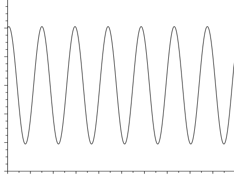
FIGURA 7. Componente x(t) de la solución del oscilador armónico con m = 2, k = 1,5, c = 0, x(0) = 10 e y(0) = 0,5 .
