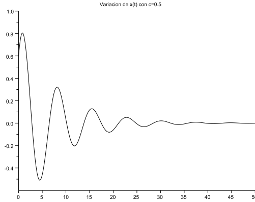
FIGURA 3. Componente x(t) de la solución del oscilador subamortiguado con m = 2, k = 1,5, c = 0,5, x(0) = 0,6 e y(0) = 0,5 .
