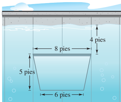
a) Compuerta de una presa
