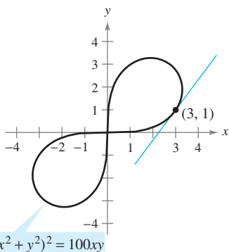
Lemniscata Figura 2.30
