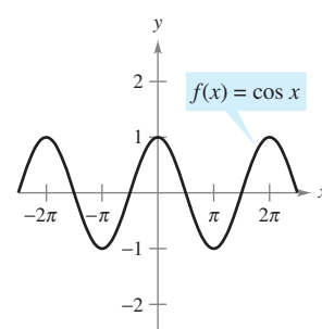
Función coseno
