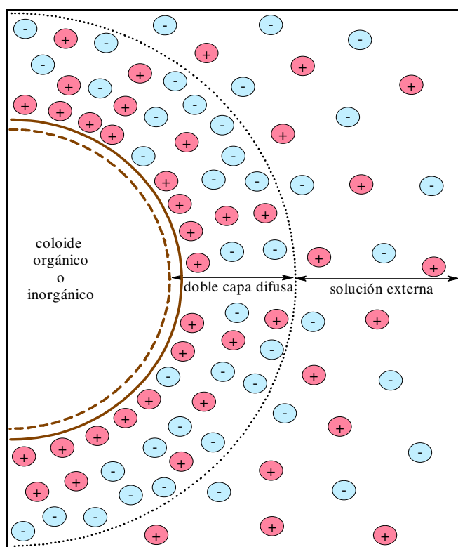
Figura 12. Representación de la superficie de un coloide orgánico o inorgánico cargado negativamente y los iones que lo rodean.
