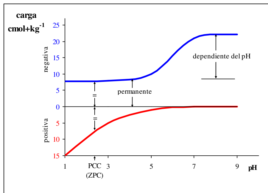
Figura 10. Esquema de la relación entre pH, cargas positivas y negativas de los coloides de un suelo.
