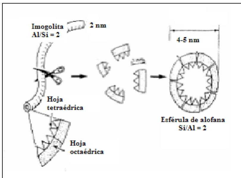
Figura 7. Diagrama esquemático de dos materiales volcánicos con estructuras atómicas similares pero diferente morfología: imogolita y alofana.
