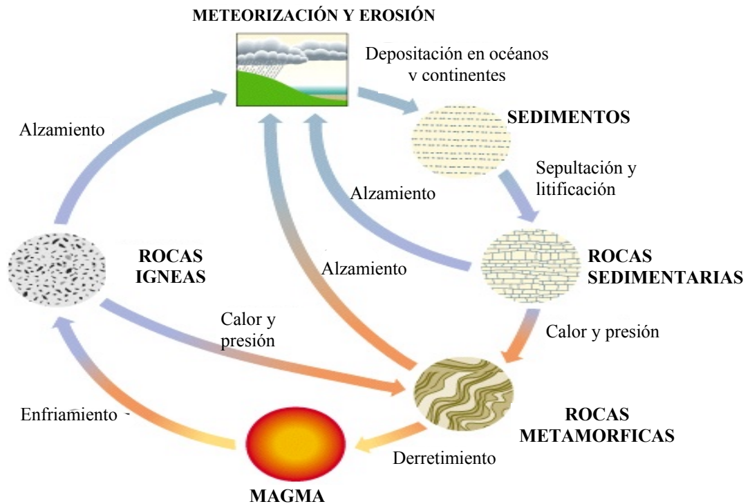
Figura 10. Ciclo de las rocas.
